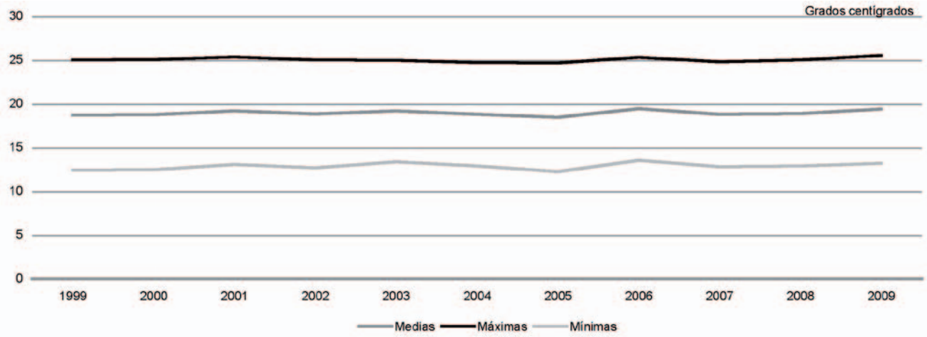
Gráfico 2.7.3 y 2.7.4. Temperaturas medias anuales en Murcia. 1999-2009
