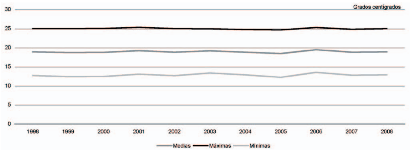
Gráfico 2.7.1 y 2.7.2. Temperaturas medias anuales en Murcia. 1998-2008
