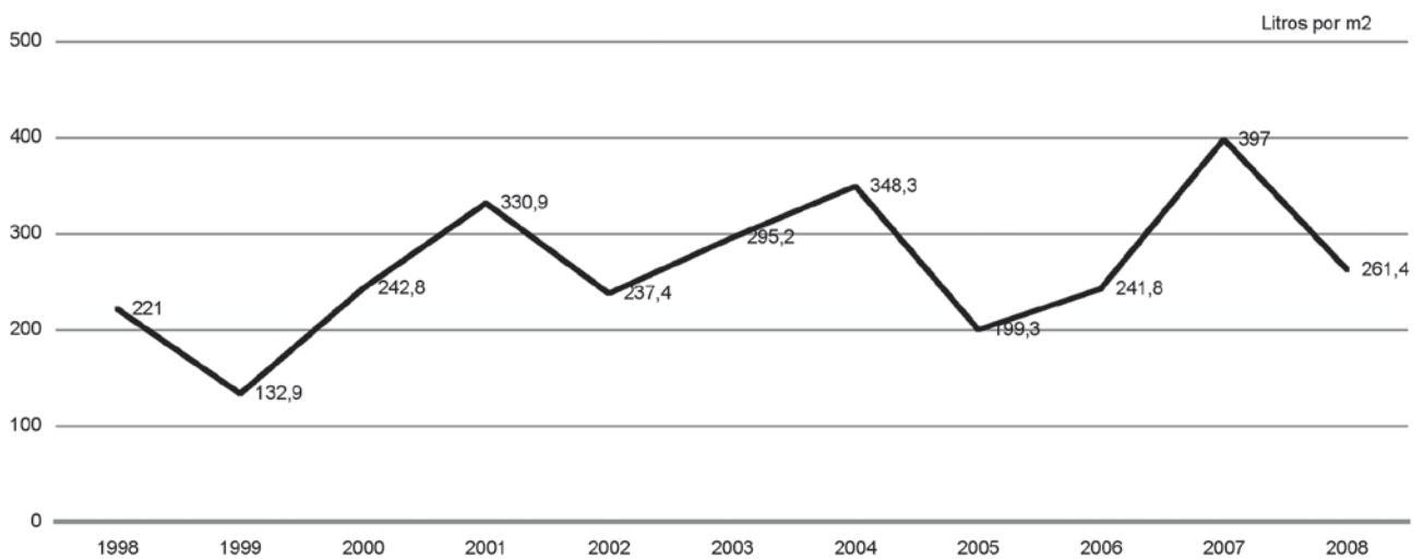
Gráfico 2.7.1 y 2.7.2. Precipitaciones totales anuales en Murcia. 1998-2008
