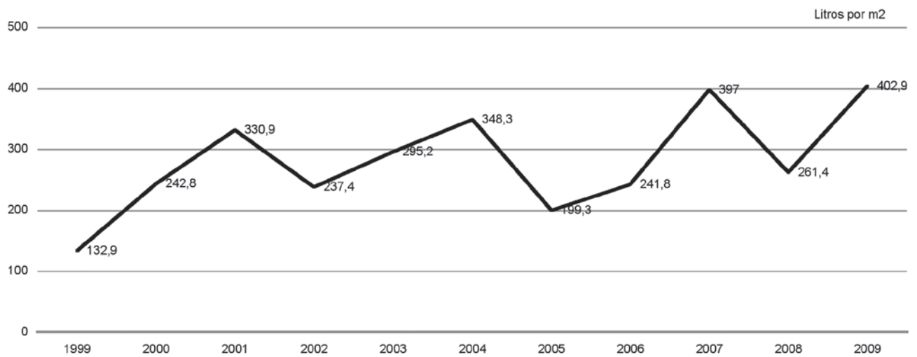
Gráfico 2.7.3 y 2.7.4. Precipitaciones totales anuales en Murcia. 1999-2009
