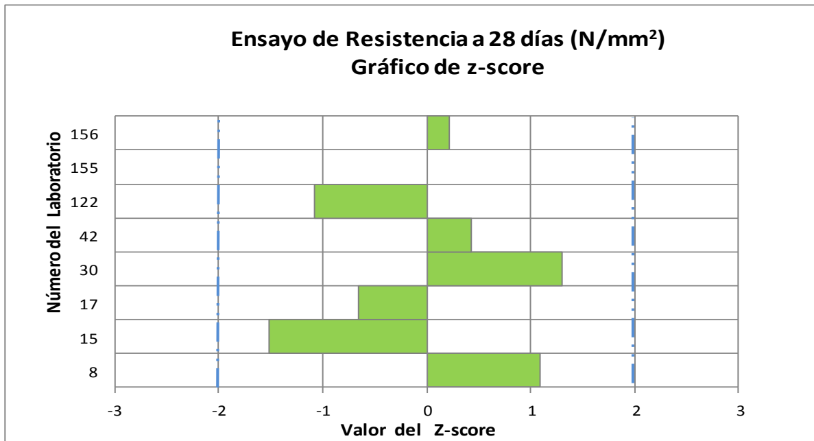
Gráfico 19. Valores de z-score Resistencia a 28 días de los laboratorios participantes de la Central de Murcia
