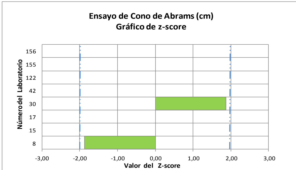
Gráfico 120. Valores de z-score del ensayo de Cono de Abrams de la Central de Murcia
