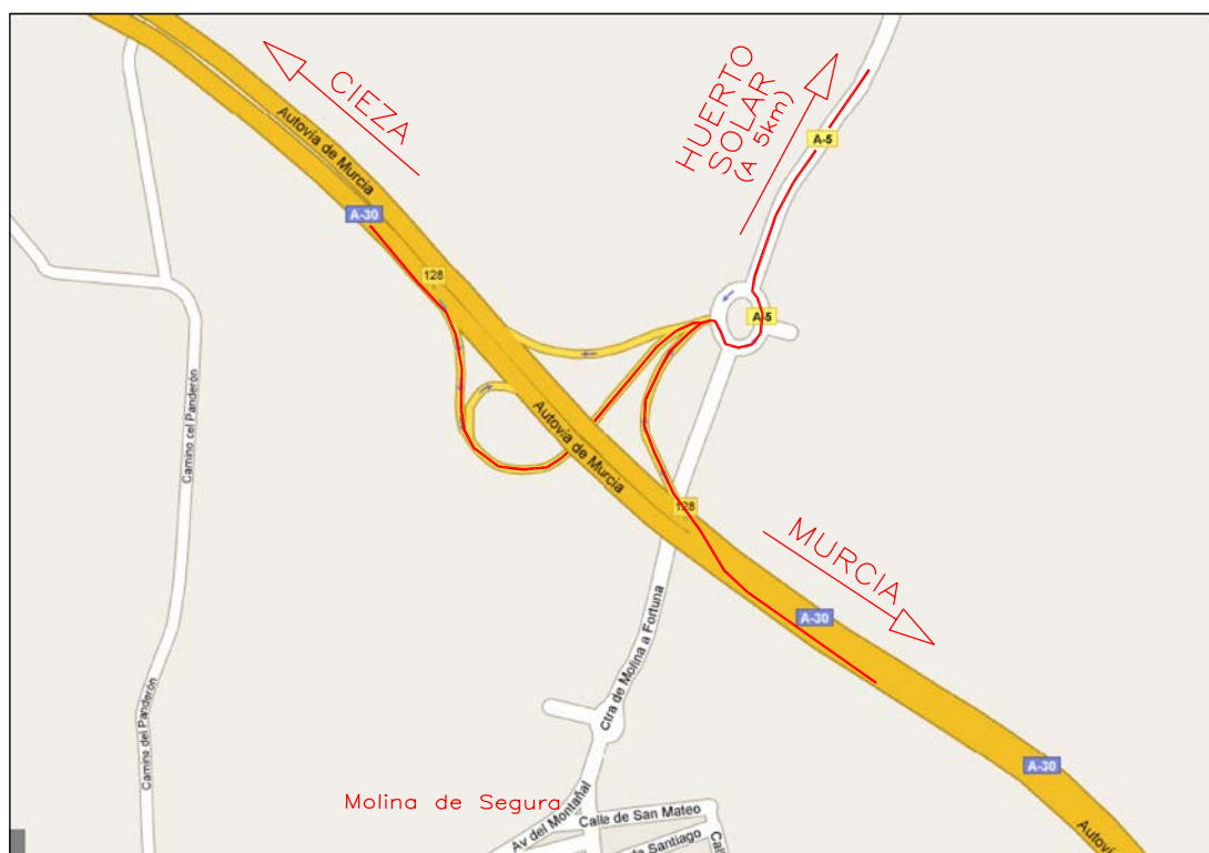
DETALLE SALIDA 128
