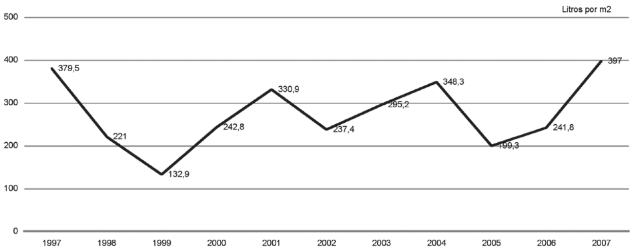
Gráfico 2.7.3 y 2.7.4. Precipitaciones totales anuales en Murcia. 1997-2007
