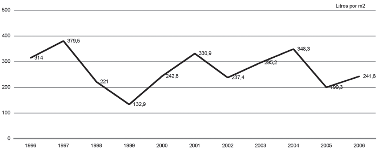
Gráfico 2.7.1 y 2.7.2. Precipitaciones totales anuales en Murcia. 1996-2006
