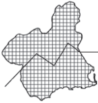
Gráfico 2.7.3 y 2.7.4. Temperaturas medias anuales en Murcia. 1997-2007
