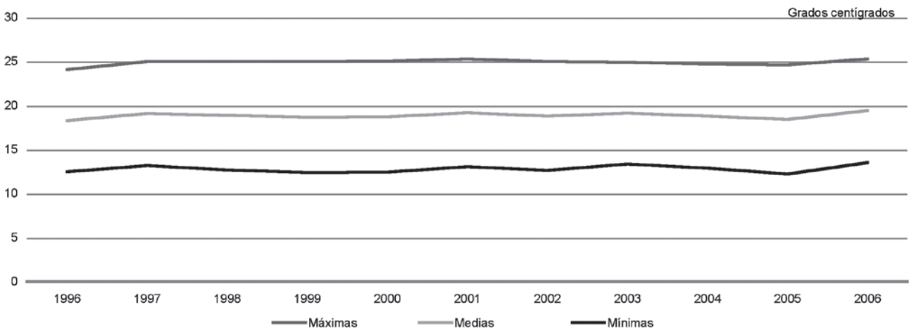
Gráfico 2.7.1 y 2.7.2. Temperaturas medias anuales en Murcia. 1996-2006
