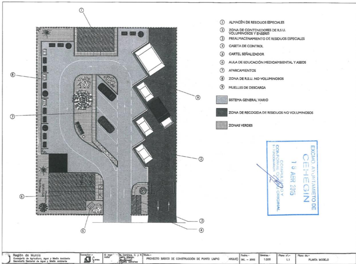
Fig. 1. Planta del ecoparque de Cehegín (Fuente: Proyecto)
