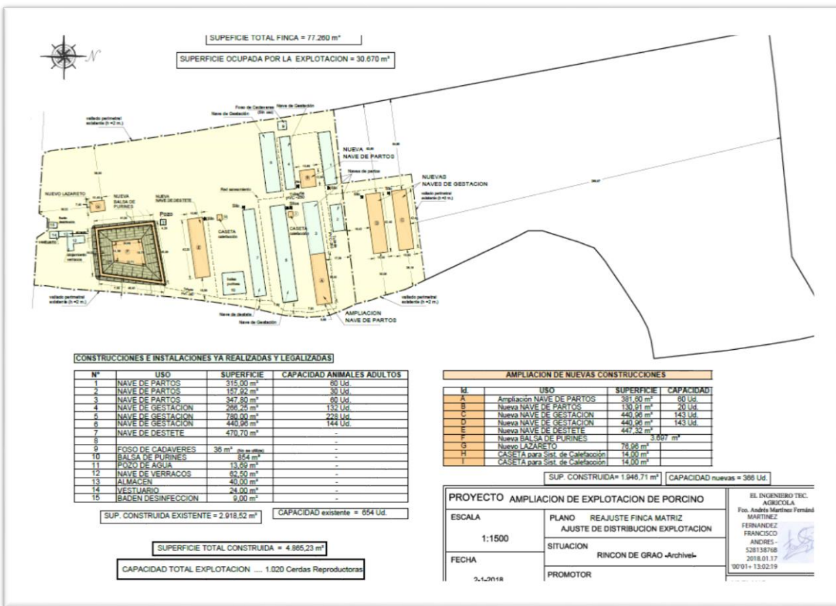
Plano en planta de las instalaciones existentes y proyectadas
