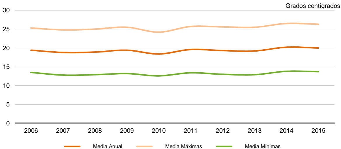
Gráfico 2.7.3.a Temperaturas medias anuales en Murcia. 2006-2015
