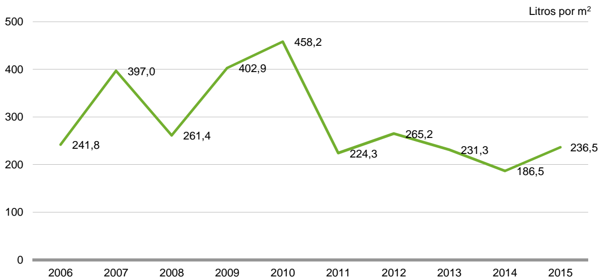
Gráfico 2.7.3.b Precipitaciones totales anuales en Murcia. 2006-2015
