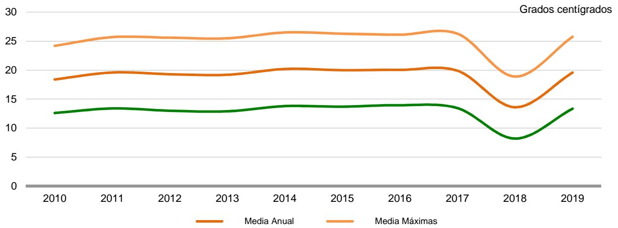
Gráfico 2.7.2.a Temperaturas medias anuales en Murcia. 2010-2019
