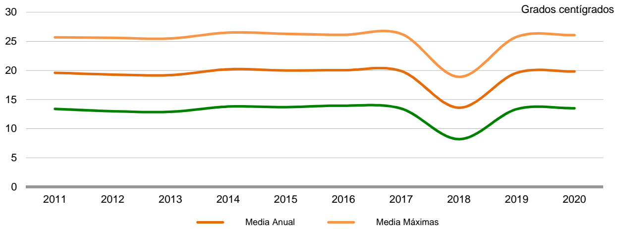
Gráfico 2.7.4.a Temperaturas medias anuales en Murcia. 2011-2020
