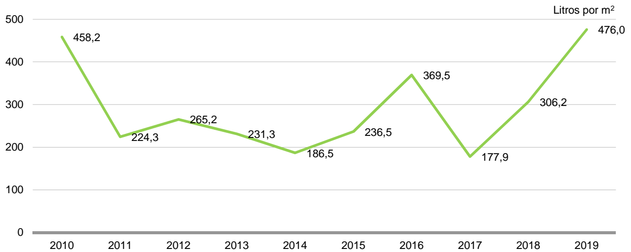
Gráfico 2.7.2.b Precipitaciones totales anuales en Murcia. 2010-2019
