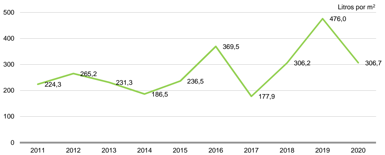
Gráfico 2.7.4.b Precipitaciones totales anuales en Murcia. 2011-2020
