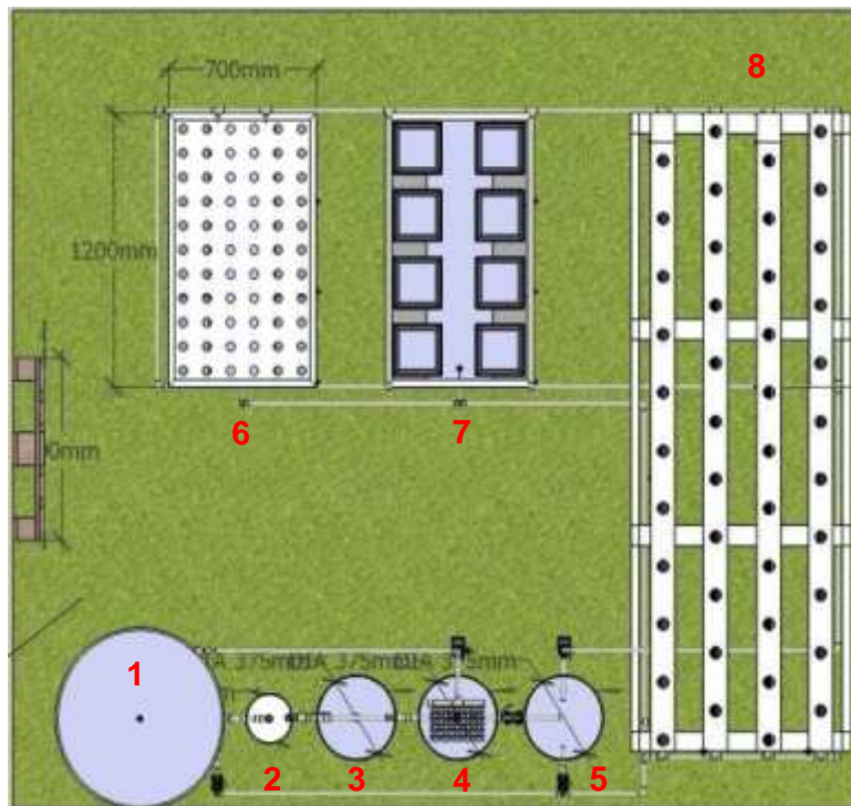
Figura 3: Componentes de la instalación de Acuaponía
