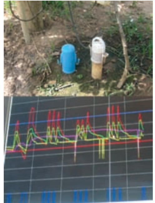
Sondas FDR que hacen la lectura de humedad en el suelo. Los datos recogidos a distintas profundidades se reflejan con varias gráficas en la pantalla del ordenador, desde donde se programa el riego.
