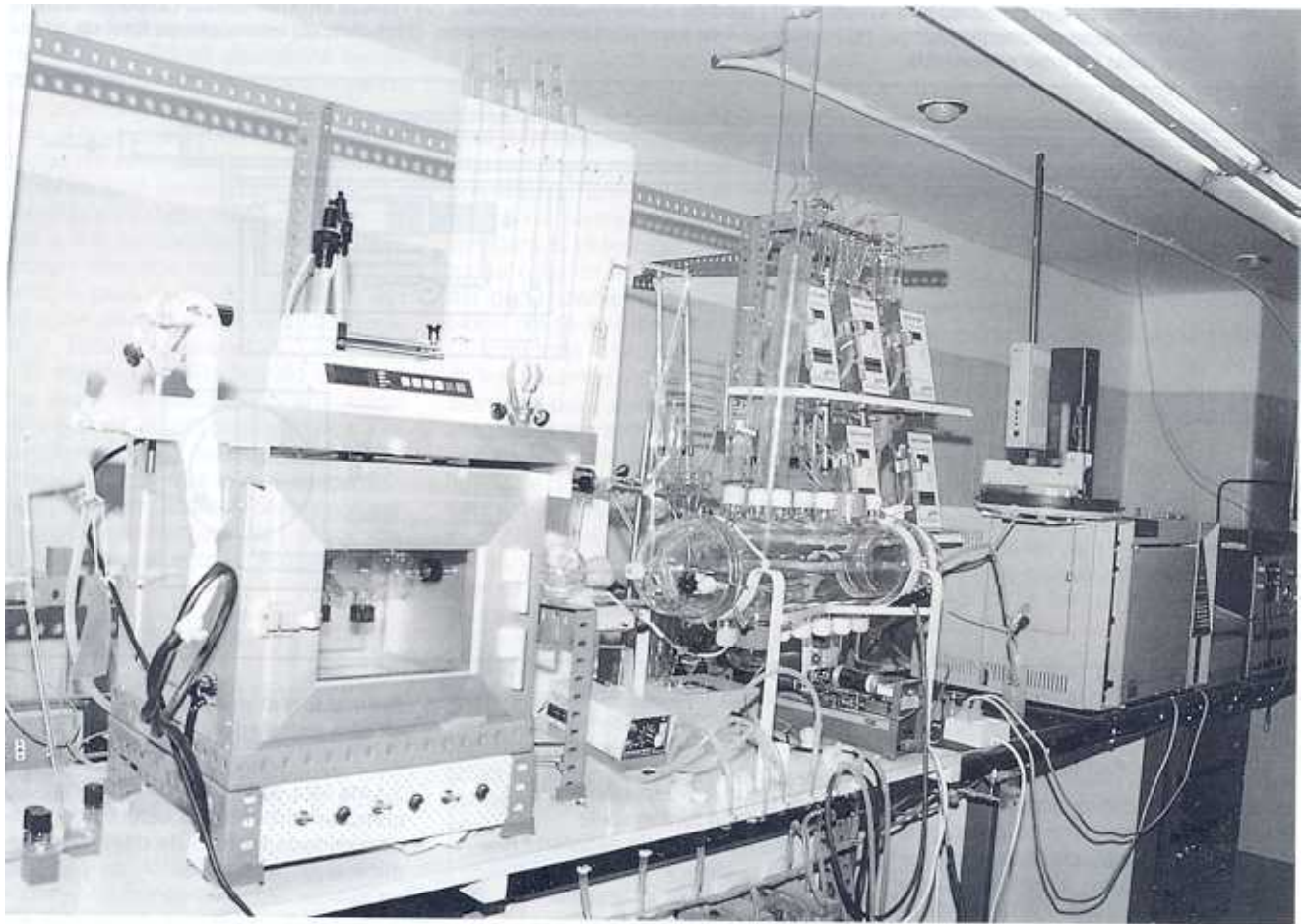
Instalación de atmósfera controlada.
