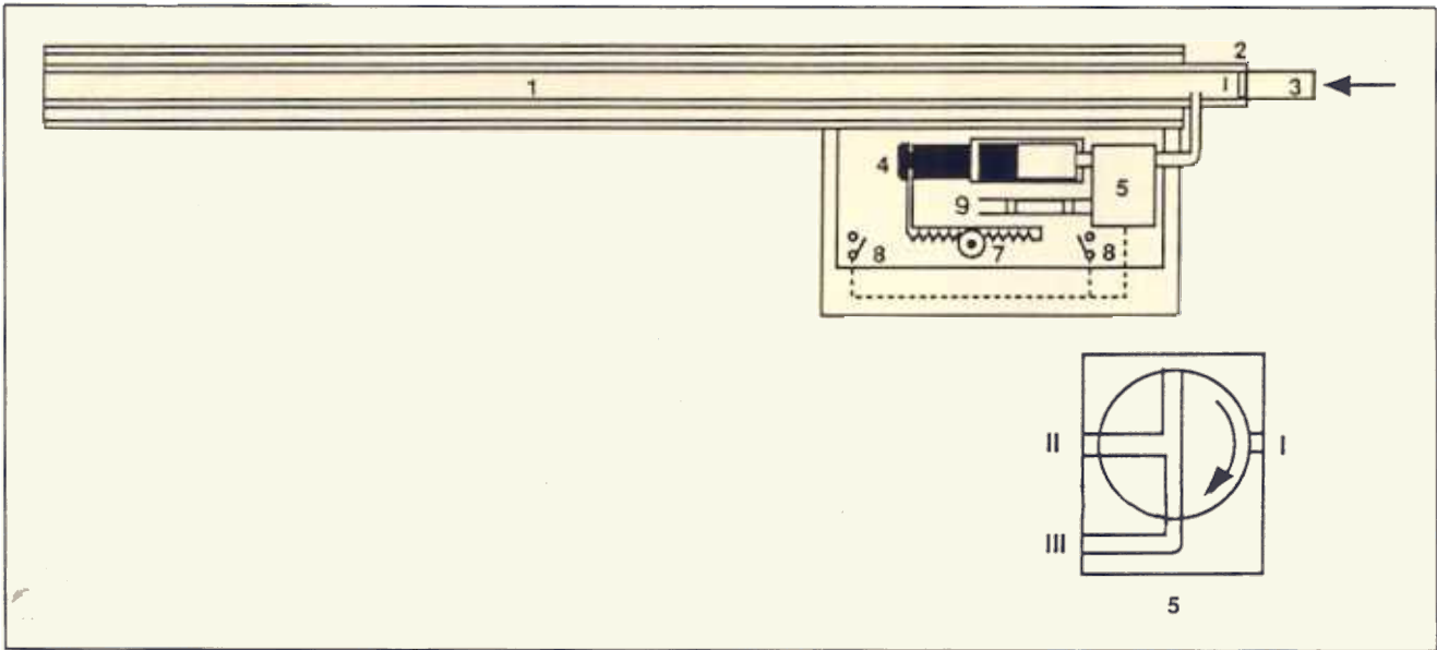
FIGURA Sistema de captación de aire exhalado: (1) tubo de aluminio calorifugado; (2) válvula antirretroceso; (3) boquilla de cartón desechable; (4) jeringa; (5) válvula de tres vías; (6) tubo adsorbente; (7) motor; (8) interruptores final de carrera; (9) tubo adsorbente.
