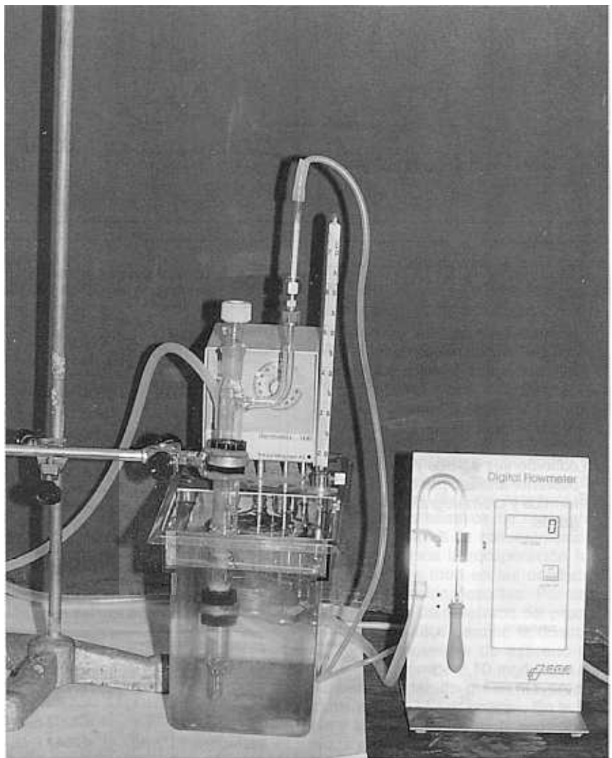
Sistema de purga y trampa.
